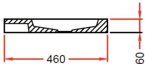
Doorsnede
