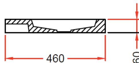
Doorsnede
